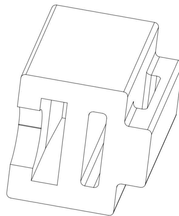
轴测图 比例 4:1
